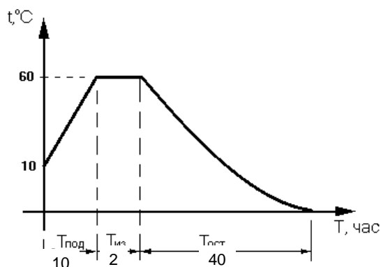
Рисунок К.1 – Температурный режим твердения бетона
