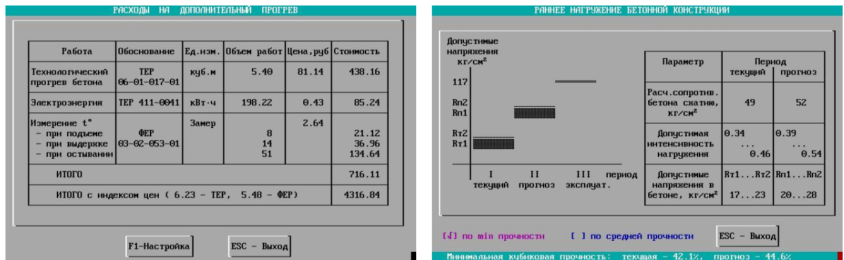
Рисунок Л.7 – Расчёт технико-экономических показателей и параметров раннего нагружения
