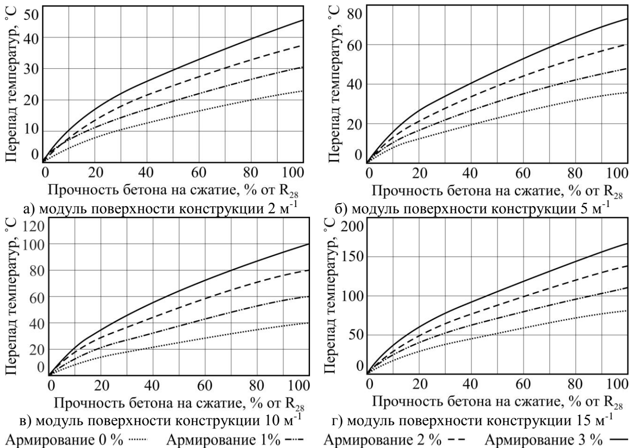
Рисунок 17.3 – Максимально допустимые перепады температур между поверхностью бетона и окружающим воздухом при распалубке
