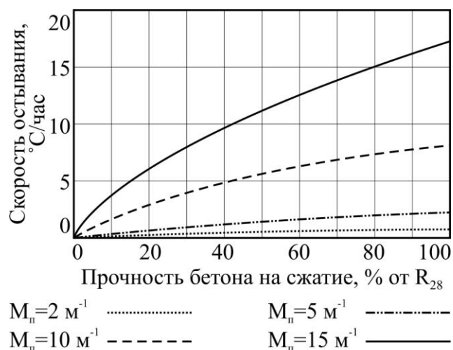
Рисунок 17.1 – Максимально допустимые скорости остывания бетона
