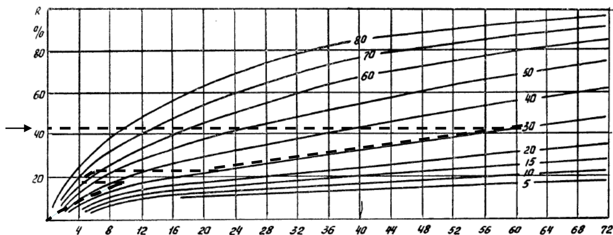
Рисунок К.2. Температурный график
