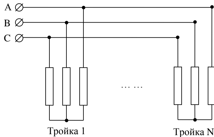
Рисунок 7.1 – Схема соединения проводов звездой
