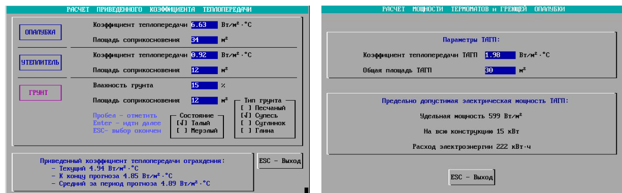
Рисунок Л.4 – Расчёт приведённого коэффициента теплопередачи ограждения и мощности поверхностных нагревателей
