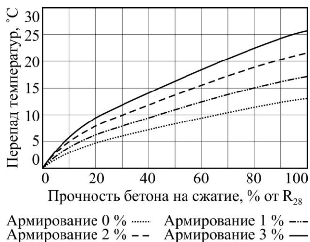
Рисунок 17.2 – Максимально допустимые скорости остывания бетона
