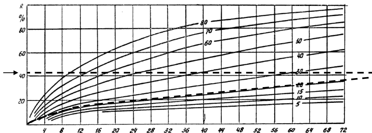
Рисунок К.3. Температурный график
