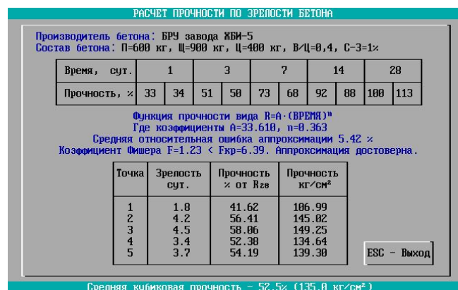
Рисунок Л.2 – Контроль параметров зимнего бетонирования
